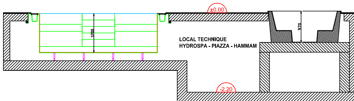
COUPE DE PRINCIPE
